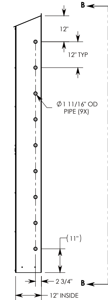
SECTION A-A
