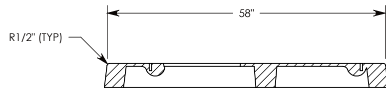
SECTION A-A
