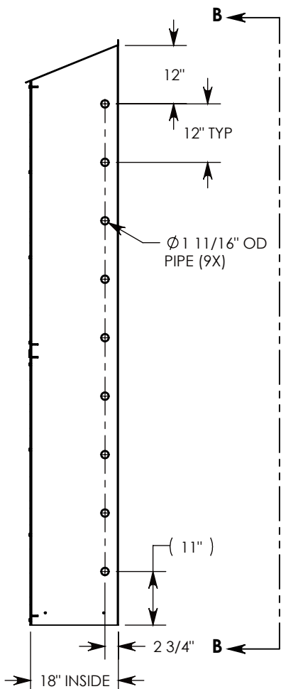
SECTION A-A
